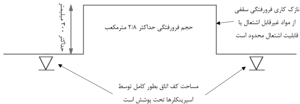
شکل ۴-۶-۱۷- شرایط عدم نصب اسپرینکلر در داخل فرورفتگی
