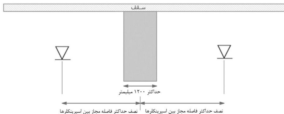
شکل ۴-۶-۱۸-ب- استثناء قانون تیر برای موانع با حداکثر عرض ۱,۲ متر
