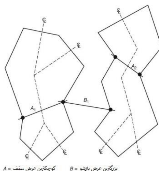
شکل ۴-۵-۱۲ ب- سقف ابری نامنظم
