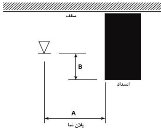
شکل ۲۱-۵-۴- فاصله اسپرینکلرها از موانع ممتد نزدیک به سقف
