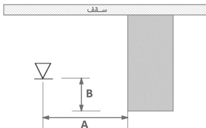
شکل ۴-۷-۴-الف- موقعیت اسپرینکلر پوشش گسترده دیواری نسبت به موانع مجاور
