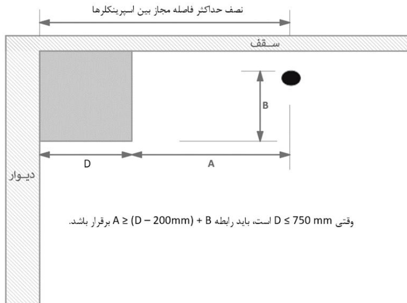
شکل ۴-۷-۴۳-ج- فاصله اسپرینکلرهای پوشش گسترده دیواری از موانع چسبیده به دیوار
