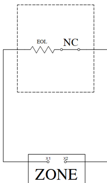
شکل پ-۸-۵- ارتباط تجهیزات سیستم اطفای با سیستم اعلام حریق متعارف - پایش خطا
