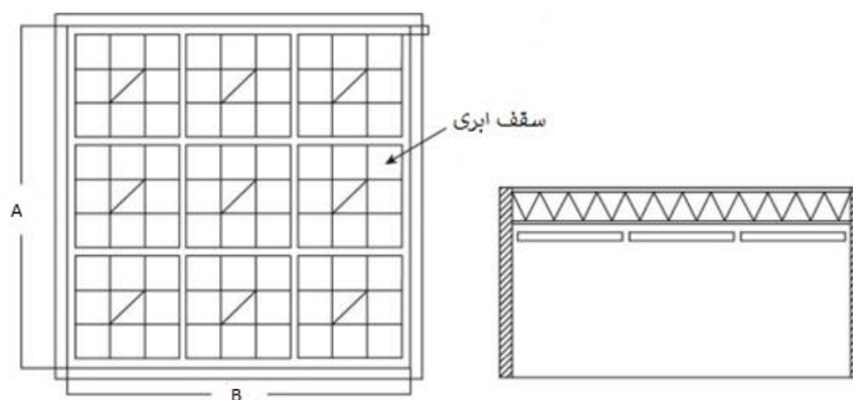
شکل ۴-۵-۱۲ الف- سقف ابری
