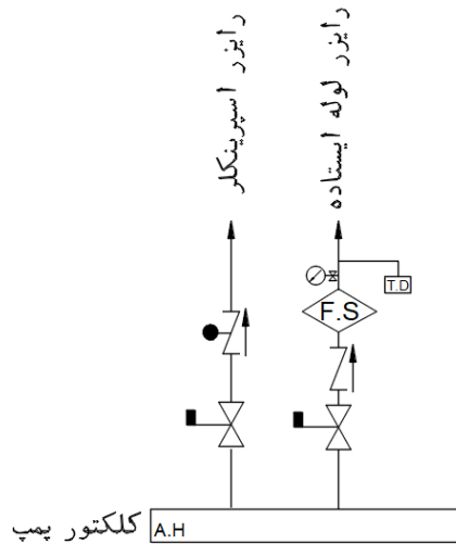
شکل پ-۲-۲- یک رایزر مستقل برای اسپرینکلر و یک رایزر مستقل برای لوله ایستاده
