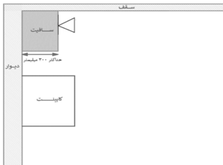
شکل ۴-۶-۲۴- عدم نیاز به نصب اسپرینکلر زیر کابینت یا ساقیت
