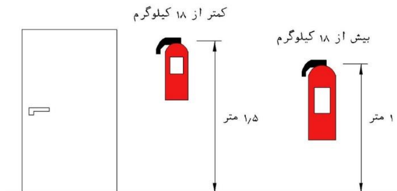
شکل ۴-۳-۸- ارتفاع نصب خاموش‌کننده دستی از کف تمام‌شده بنا
