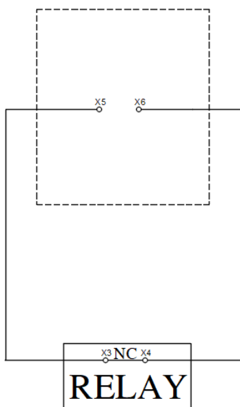
شکل پ-۸-و- ارتباط تجهیزات سیستم اطفای با سیستم اعلام حریق متعارف - خروجی فرمان
