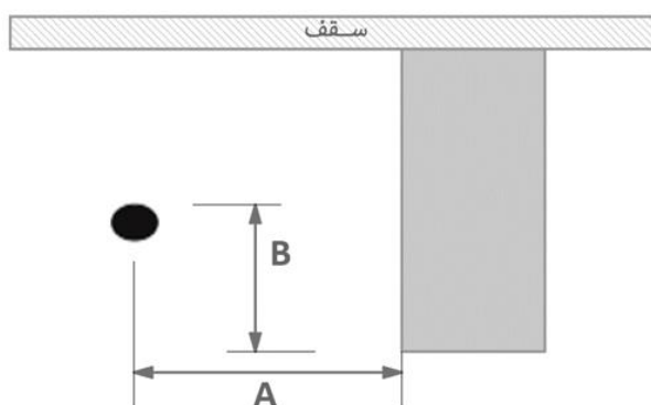
شکل ۴-۶-۲۱-الف- موقعیت اسپرینکلر دیواری مسکونی نسبت به موانع
