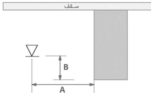
شکل ۴-۶-۱۸-الف- فاصله افقی و عمودی اسپرینکلر تا مانع
