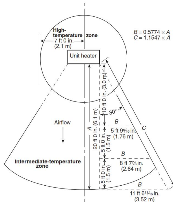
شکل ۹-۴-۴- مناطق دما بالا و دما متوسط در واحد حرارتى
