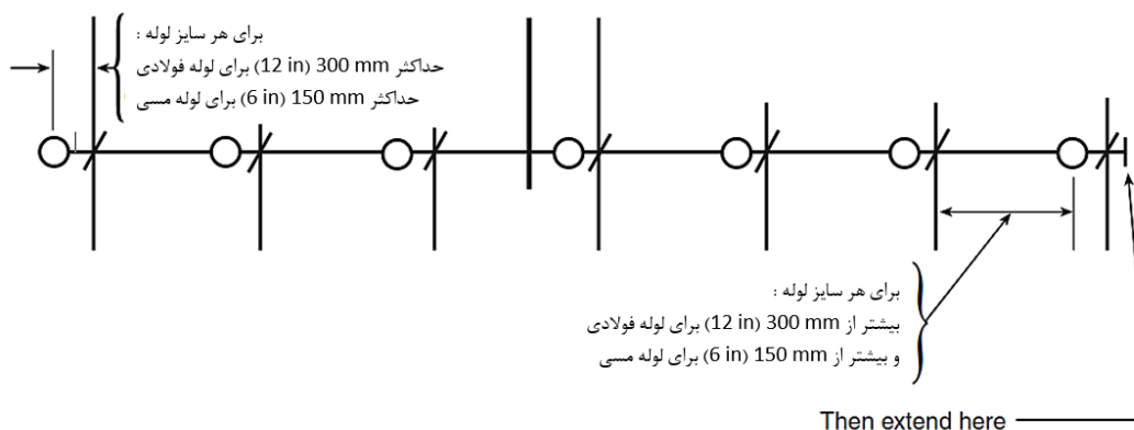
شکل پ-۶-۱۶- فاصله بین آویز و اسپرینکلر- فشار بیشتر از ۱۰۰ psi
