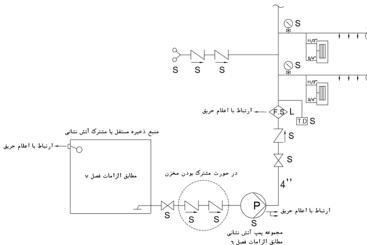
شکل پ-۱-۱- نمای شماتیک سیستم اطفای حریق S۱
