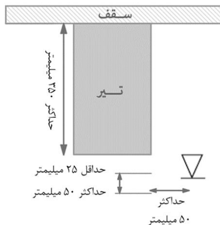
شکل ۴-۶-۹-ب- جانمایی اسپرینکلر پایین زن مسکونی در مجاورت تیر
