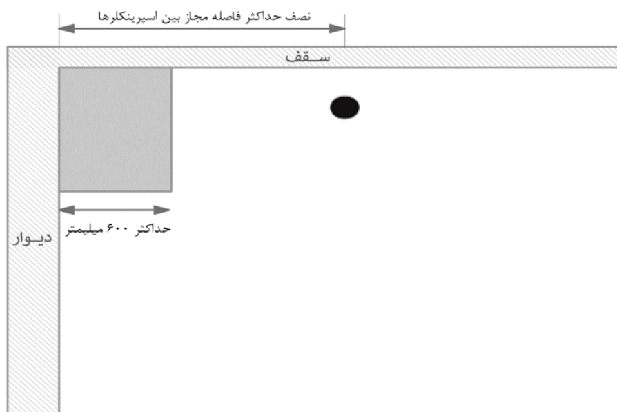
شکل ۴-۷-۴۳-د- عدم نیاز به نصب اسپرینکلر در زیر مانع چسبیده به دیوار
