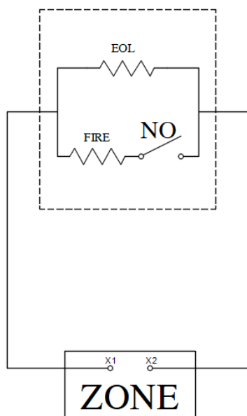
شکل پ-۸-۵- ارتباط تجهیزات سیستم اطفای با سیستم اعلام حریق متعارف- پایش حالت حریق
