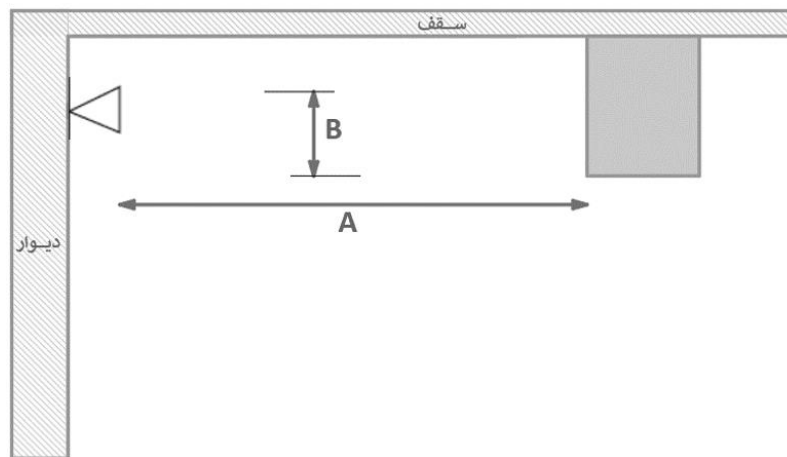
شکل ۴-۷-۴-الف موقعیت اسپرینکلر پوشش گسترده دیواری نسبت به موانع مقابل
