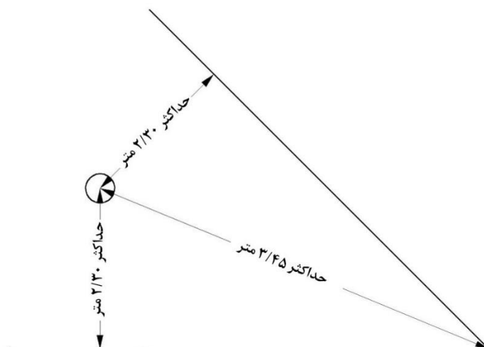
شکل ۴-۴-۱۰- حداکثر فاصله اسپرینکلر از کنج دیوار
